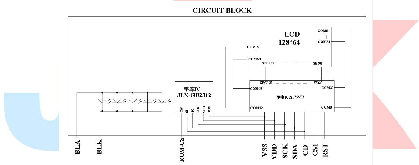
图 2: 电路框图
