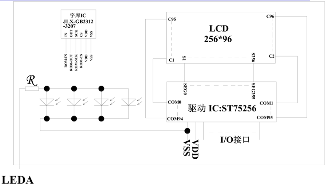
图 2: JLX25696G-967-PL 电路框图
